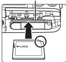
存储卡插槽
