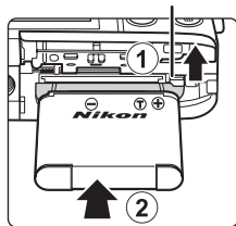
电池锁门
